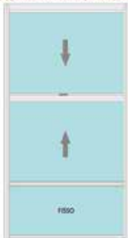
SALISCENDI MOTORIZZATA IN ALLUMINIO DUE ANTE MOBILI
